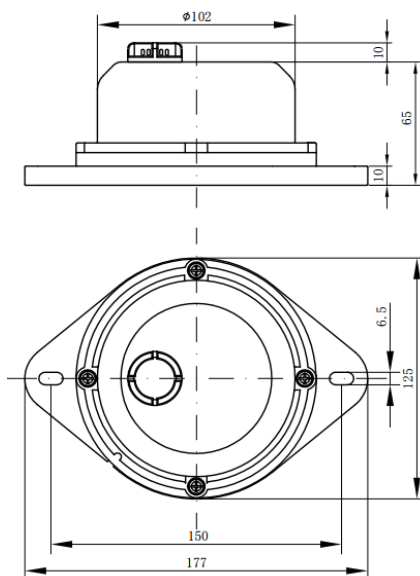
图 2 终端尺寸图
