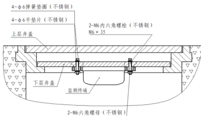
图3 双层井盖安装示意图（安装附件 CS-iTWM-08-A03）
