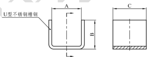
图 5 U 型槽钢加工示意图
