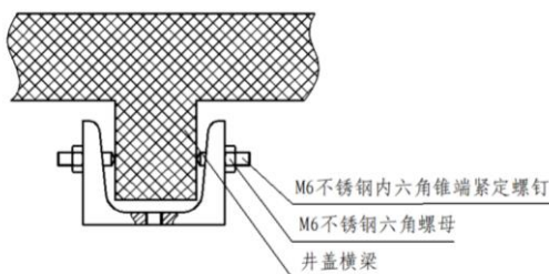
图 7 U 型槽钢安装示意图
