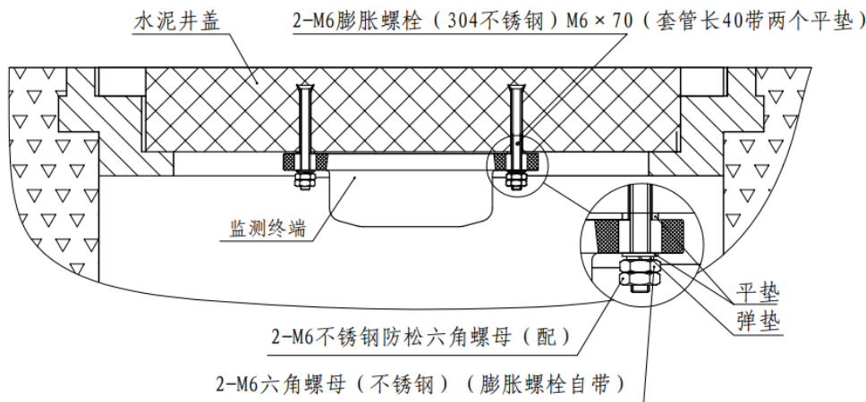
图 10 钢筋混凝土井盖安装示意图（安装附件 CS-iTWM-08-A04）
