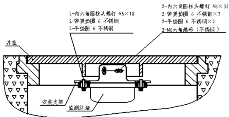
图 9 雨水球墨铸铁材料井盖安装示意图（安装附件 CS-iTWM-08-A01）
